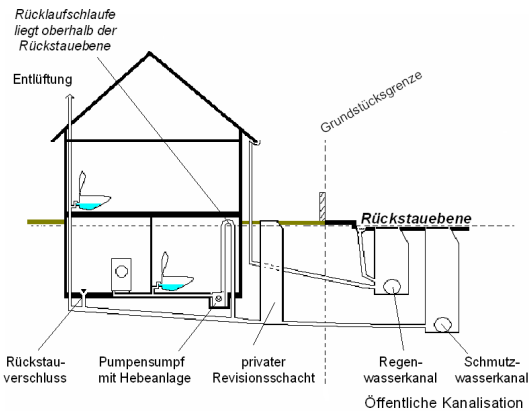
Abb. 1 - ordnungsgemäße Installation
