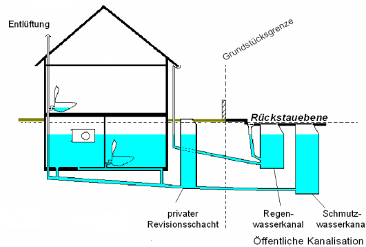
Abb. 2 - Rückstau bei fehlender Rückstausicherung
