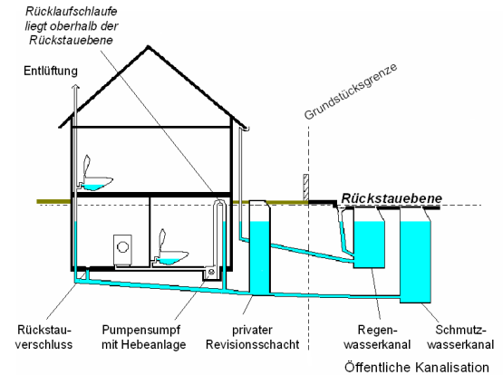
Rückstau bei funktionierender Rückstausicherung
